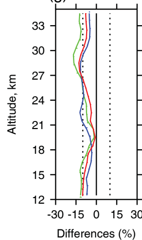
(g) 60° N–90° N
