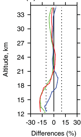
(d) 60° S–20° S
