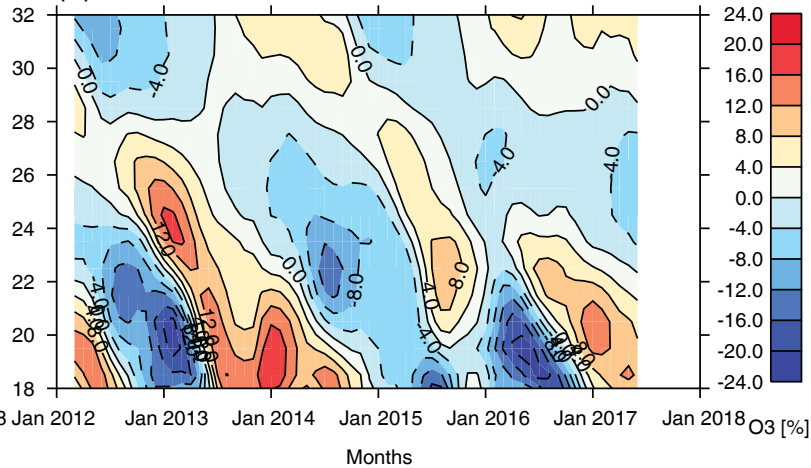
(b) Aura-MLS v4 ozone [%], 5° S–5° N
