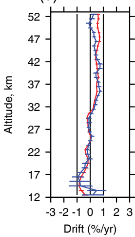
(d) 60° S–20° S
