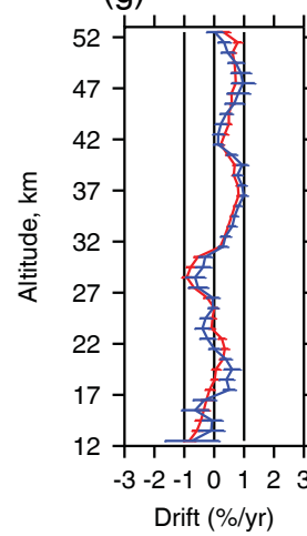
(g) 60° N–90° N
