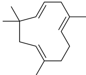
\alpha -humulene
