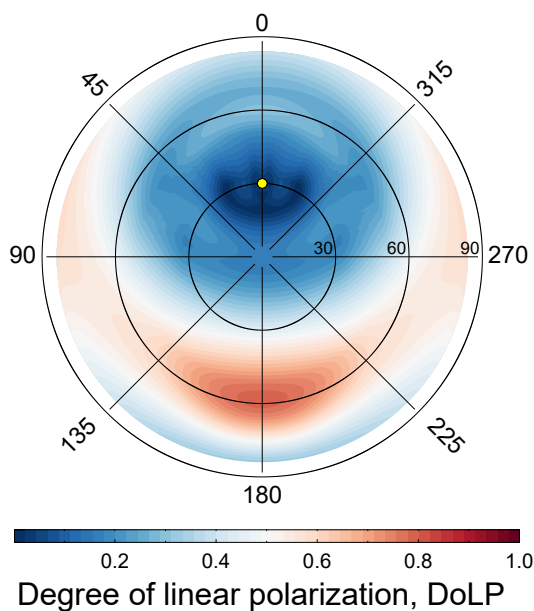
(d) BPDF (865 nm) for Maritime-ocean scene AOT (555 nm)=0.15, solar zenith angle=30°
