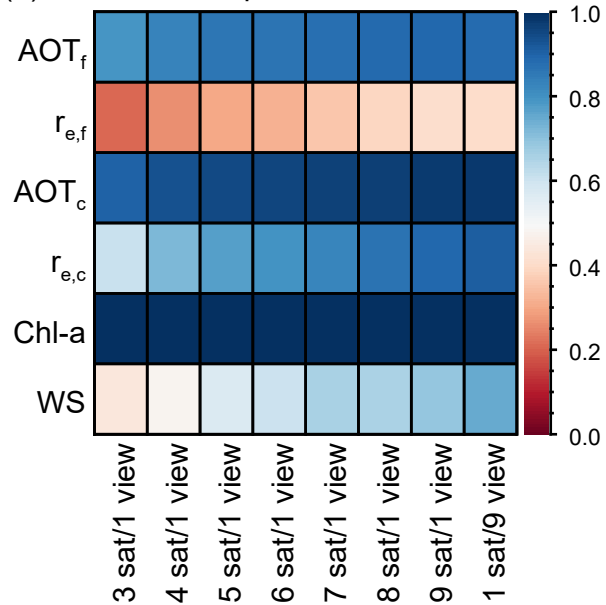
(d) Reflectance + polarization, Ocean AOT=0.1
