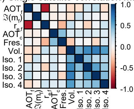
(d) Single satellite correlation matrix
