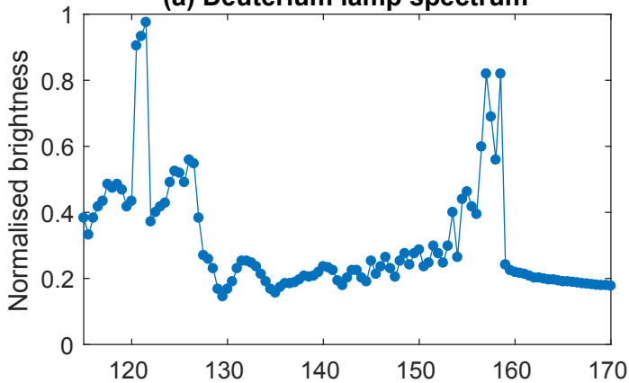
(a) Deuterium lamp spectrum
