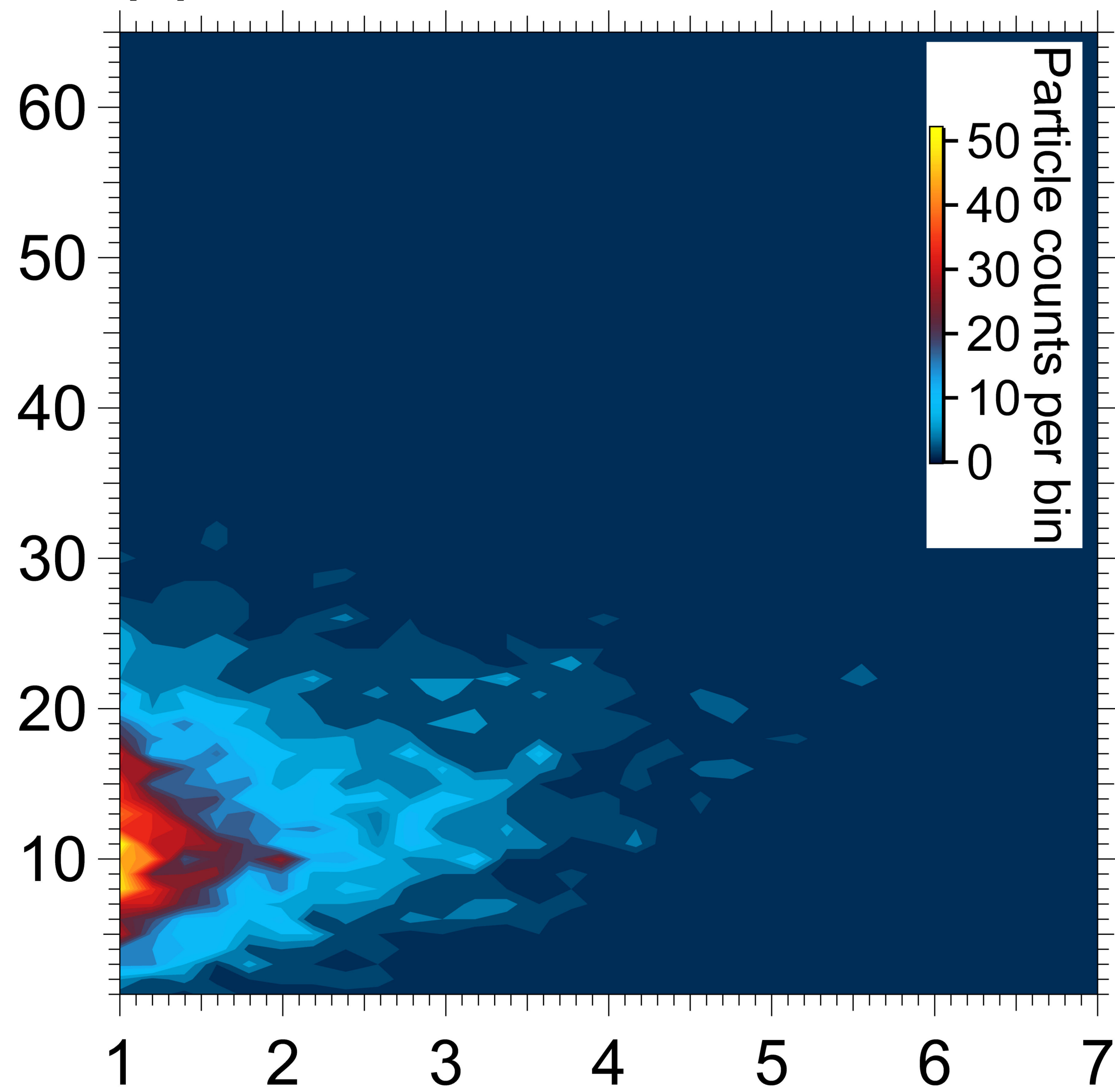
(e) \text{Fe}_3\text{O}_4
