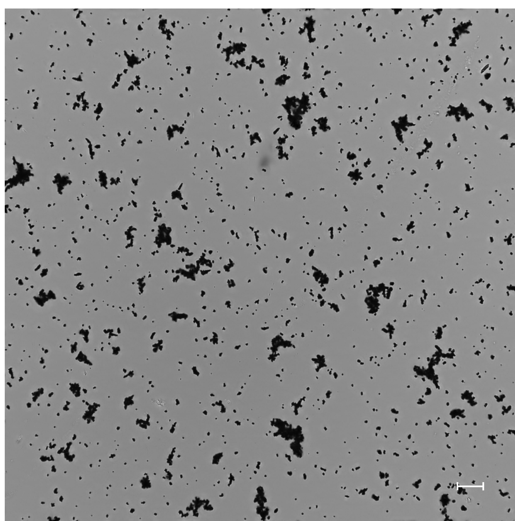
(f) \text{Fe}_3\text{O}_4
