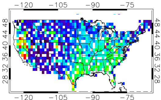
CALIOP
