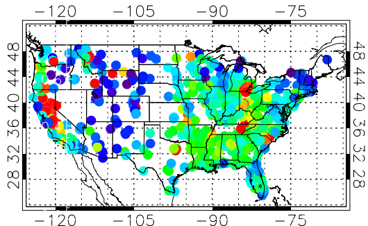
CALIOP (pairwise)
