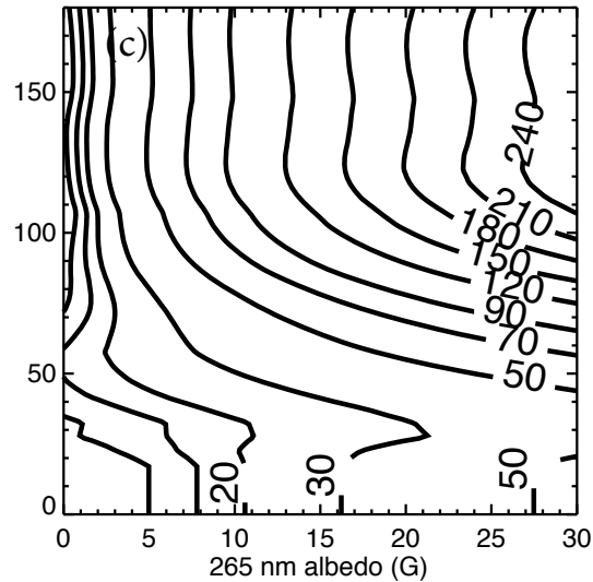
PMC IWC from AIR:CIPS
