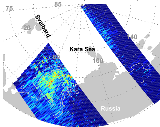
(b) OMI BrO VCD (orbit no. 73059)
