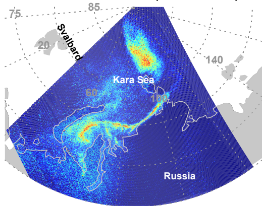
(a) TROPOMI BrO VCD (orbit no. 2537)
