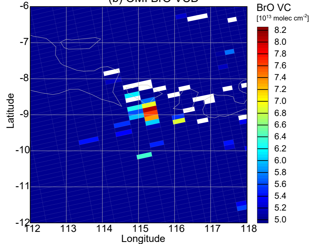
(b) OMI BrO VCD
