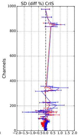
(b) CrIS
