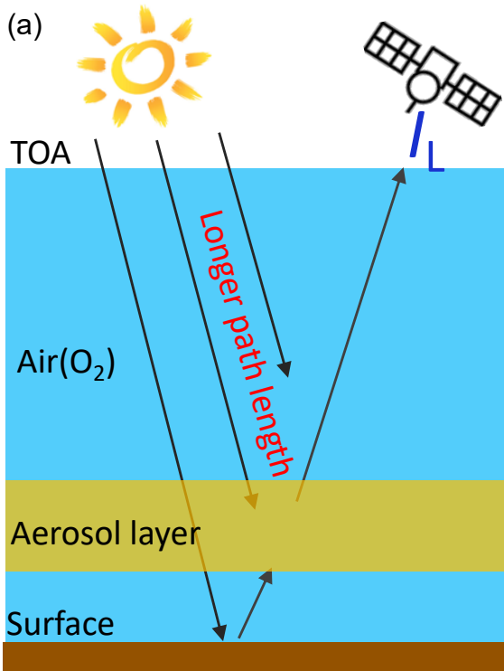
Low aerosol altitude
