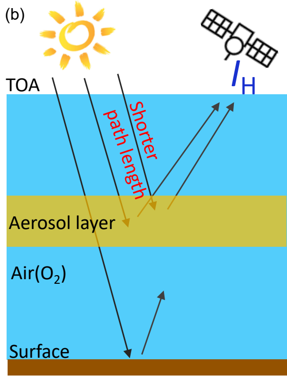
High aerosol altitude
