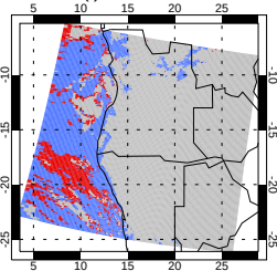
(f) COD mask
