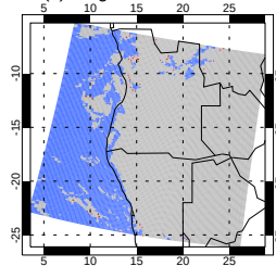
(d) Neighbour count mask
