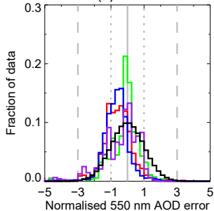
(c) VIIRS
