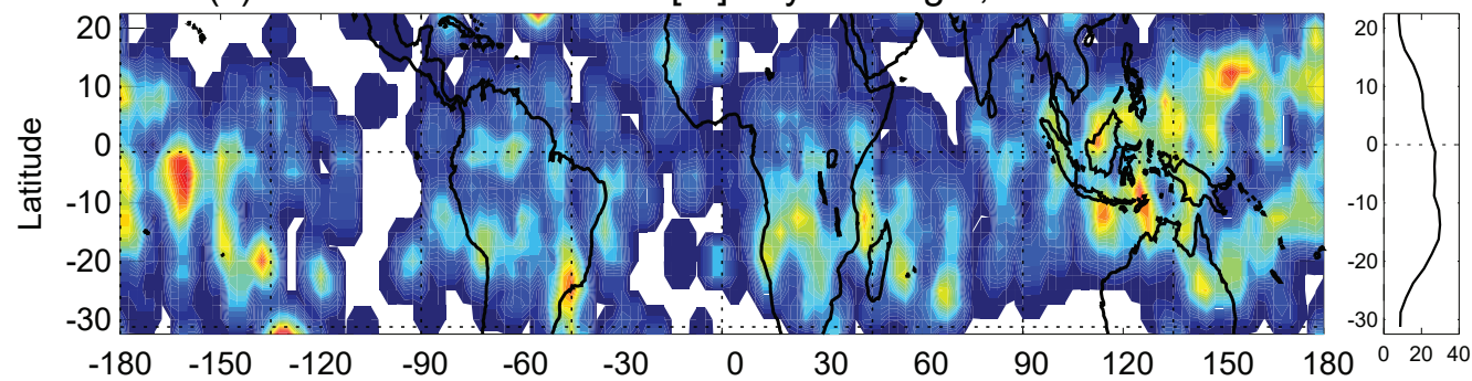
(d) CALIOP cirrus fraction [%] day and night, 25–31 Jan 2010
