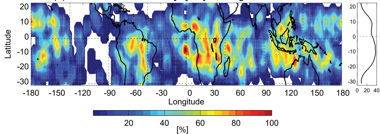
(d) CALIOP cirrus fraction [%] day and night, 25–31 Jan 2010
