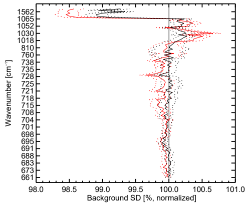
(b) CrIS
