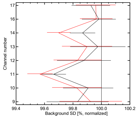
(b) CrIS
