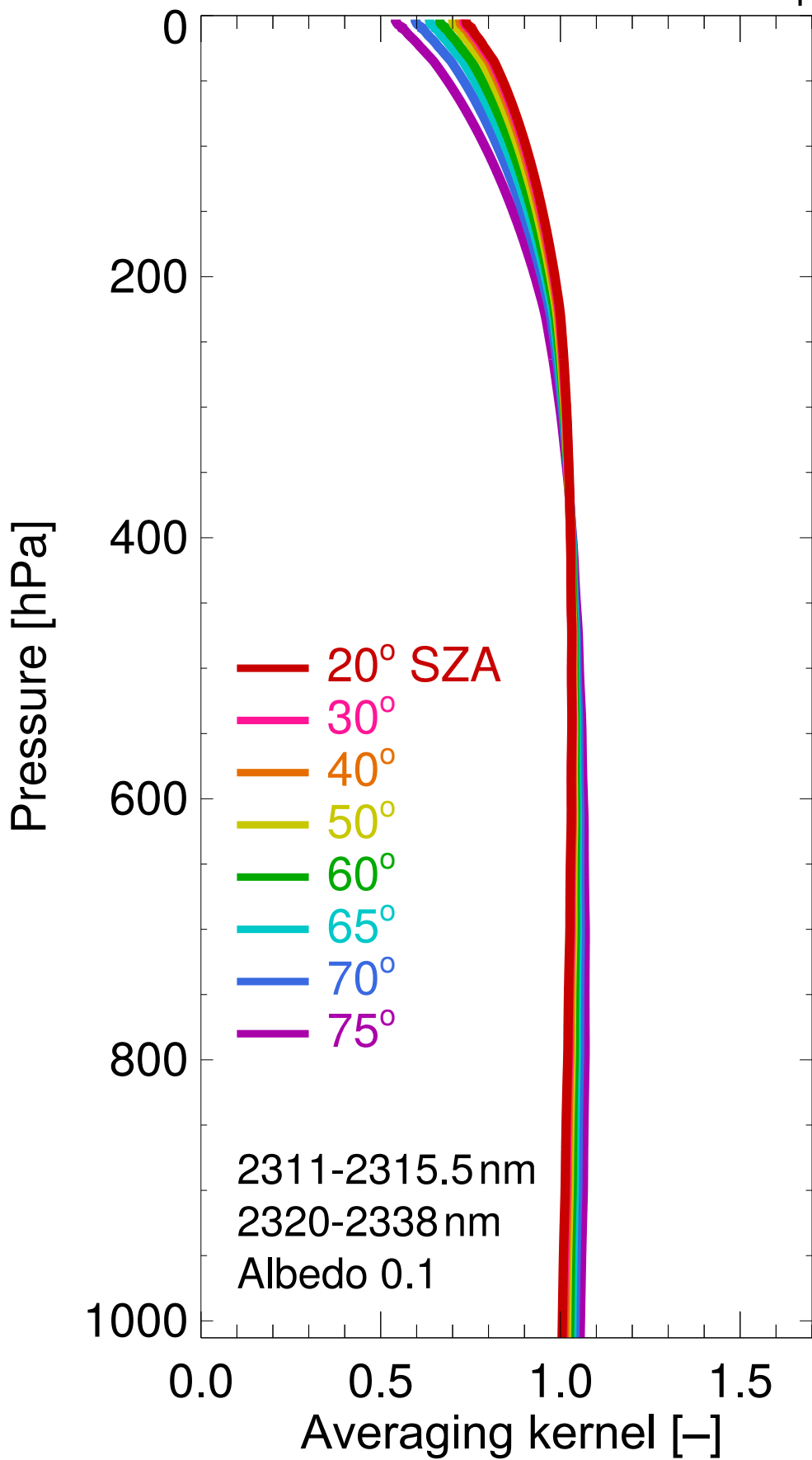
TROPOMI/WFMD CH 4
