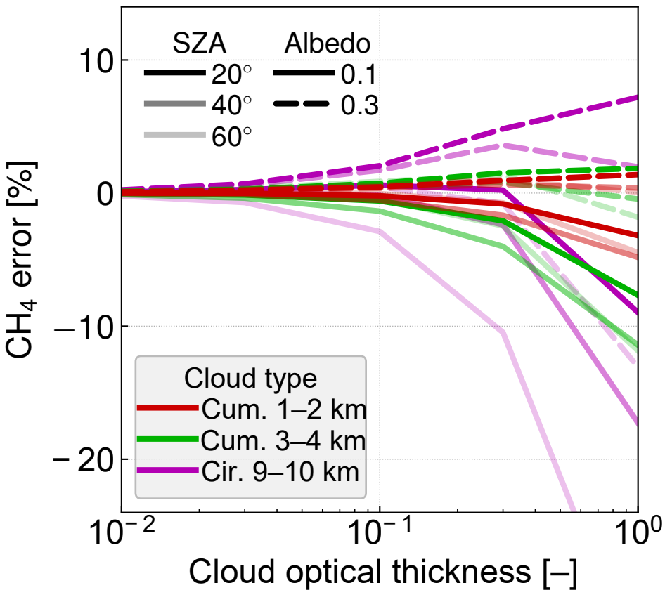
CH 4 retrieval error
