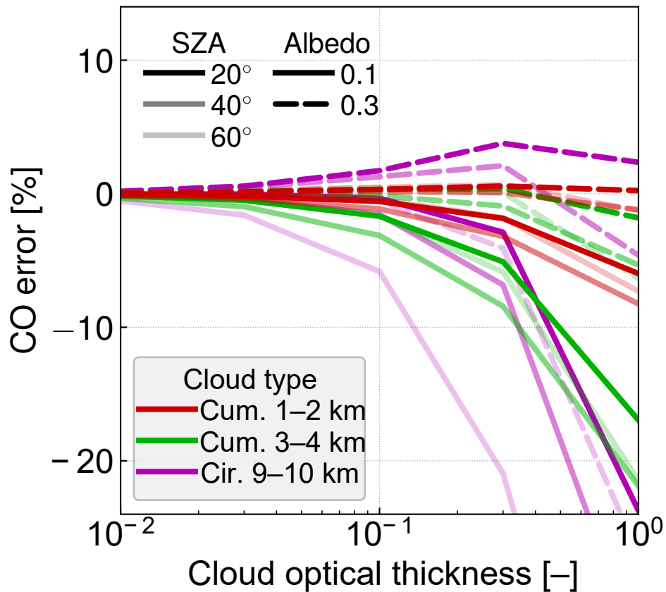
CO retrieval error
