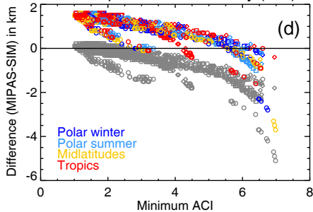
MIPAS top altitude uncertainty (ACI)
