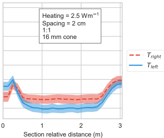
(d) Mean wind speed = 3.8 \text{ m s}^{-1}
