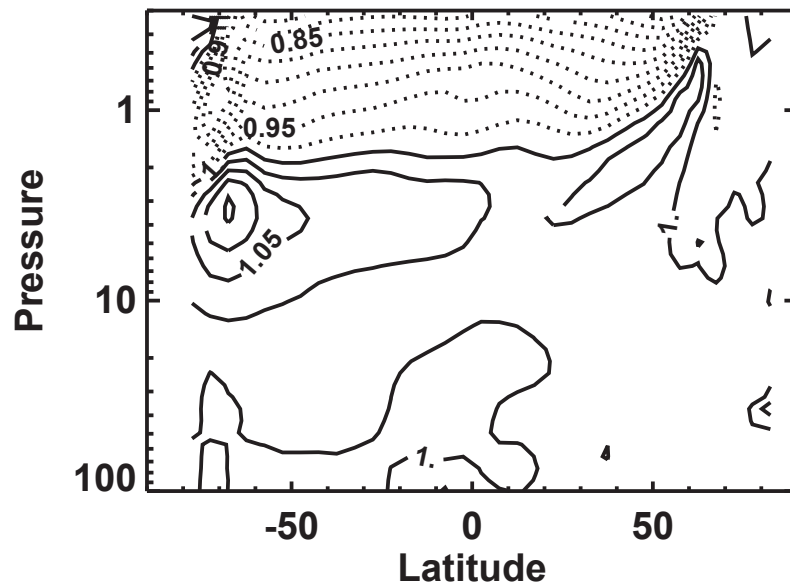
(d) Dec model ASC/DSC ratio
