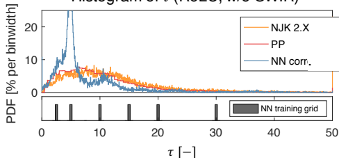
(d) Histogram of \tau (ReLU, w/o SWIR)
