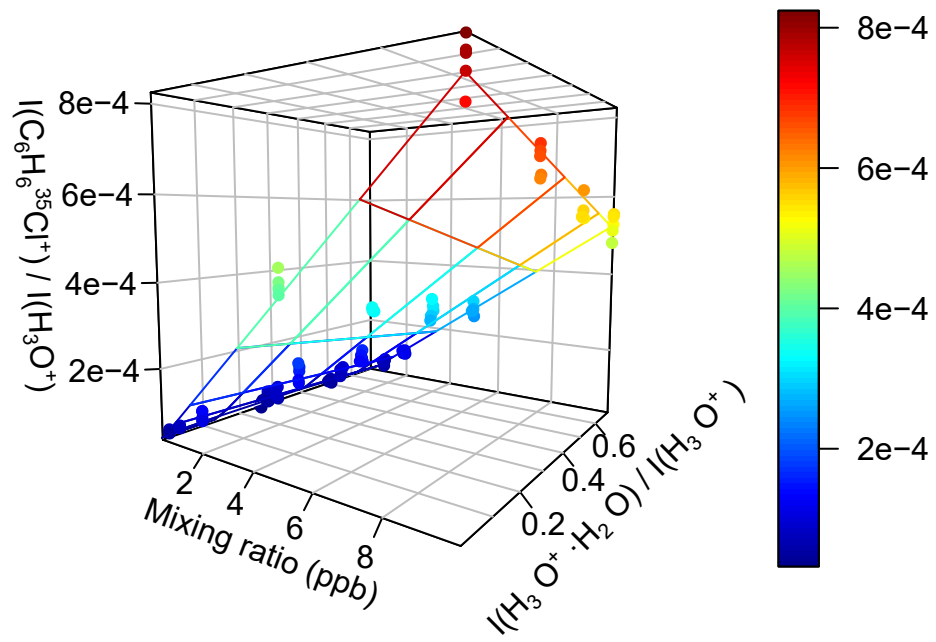
19 u / 113 u / chlorobenzene
