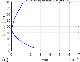
FTIR a priori profile (WACCM)
