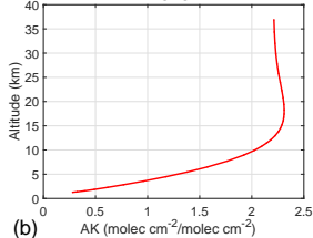
TROPOMI
