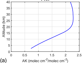
FTIR
