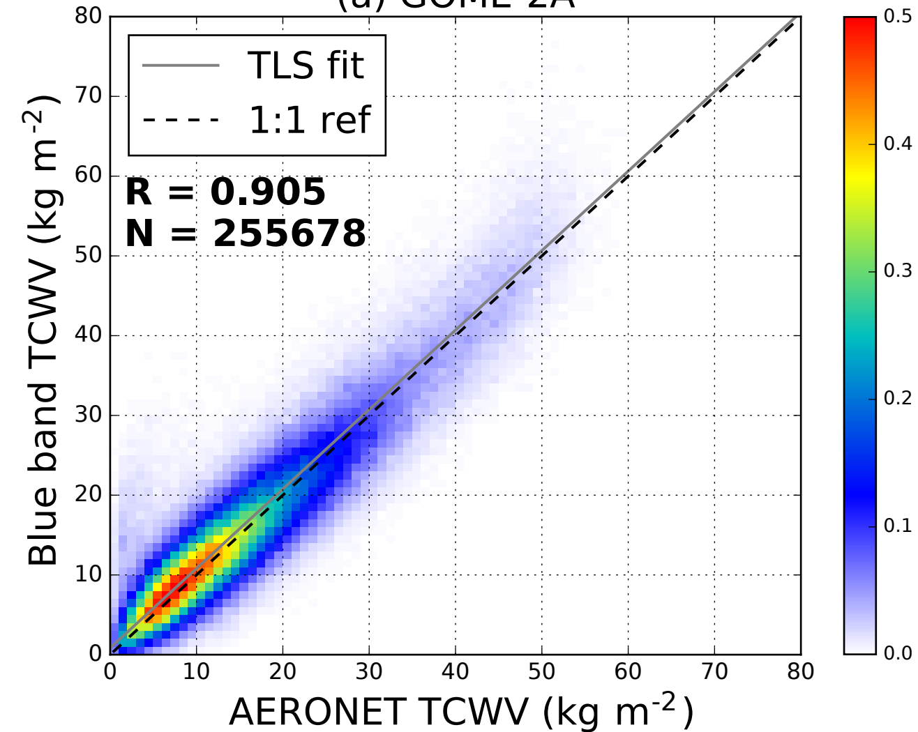
(a) GOME-2A
