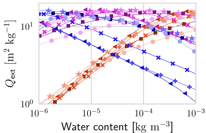
(d) 657.3 GHz
