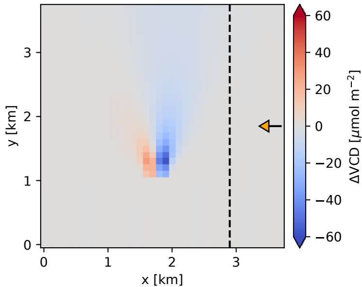
(d) \Delta VCD for SZA:40° and SAA:270°
