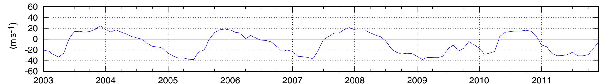
(d) Singapore monthly mean zonal wind at 10 hPa
