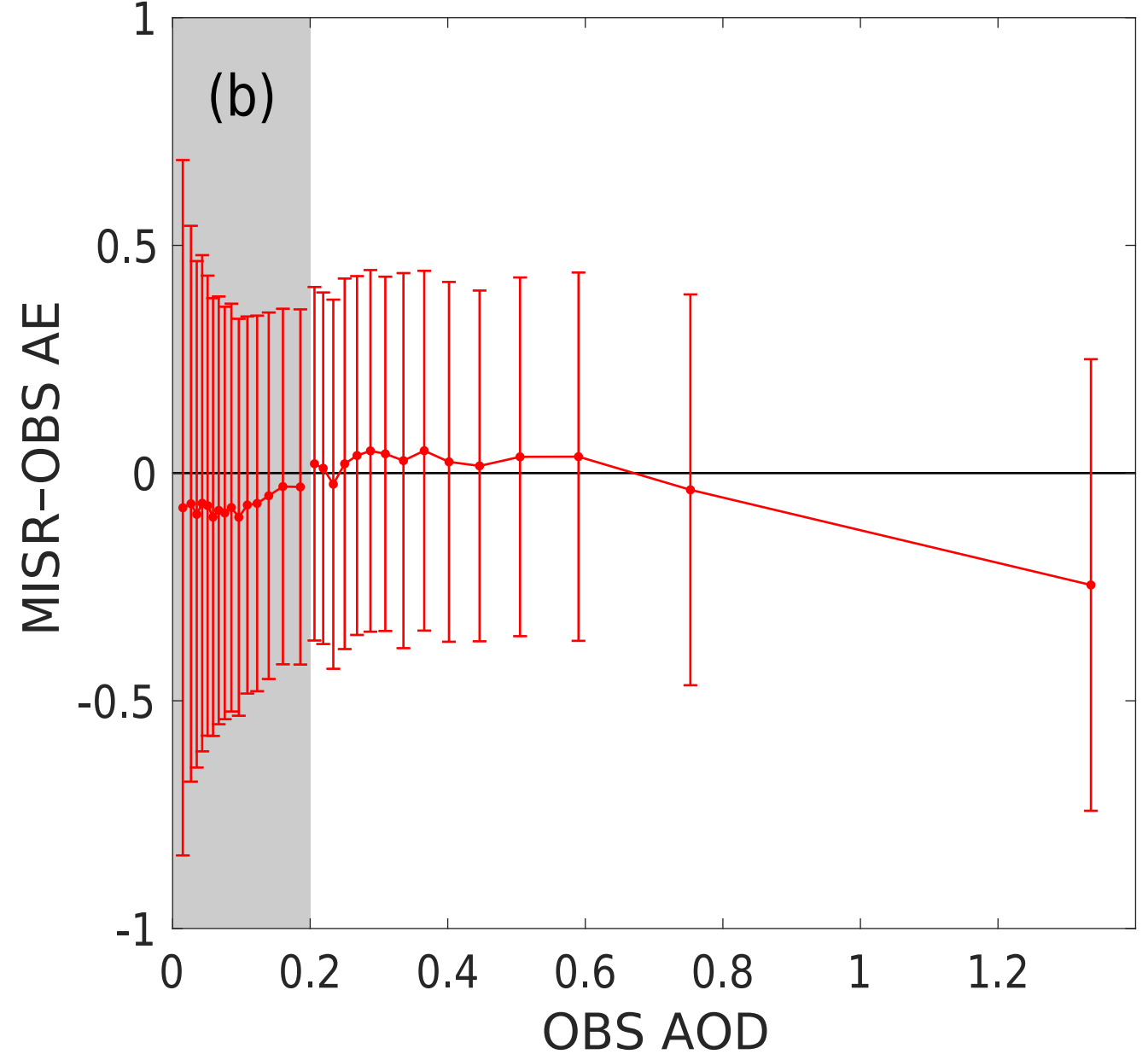
V23 AE error vs. AOD
