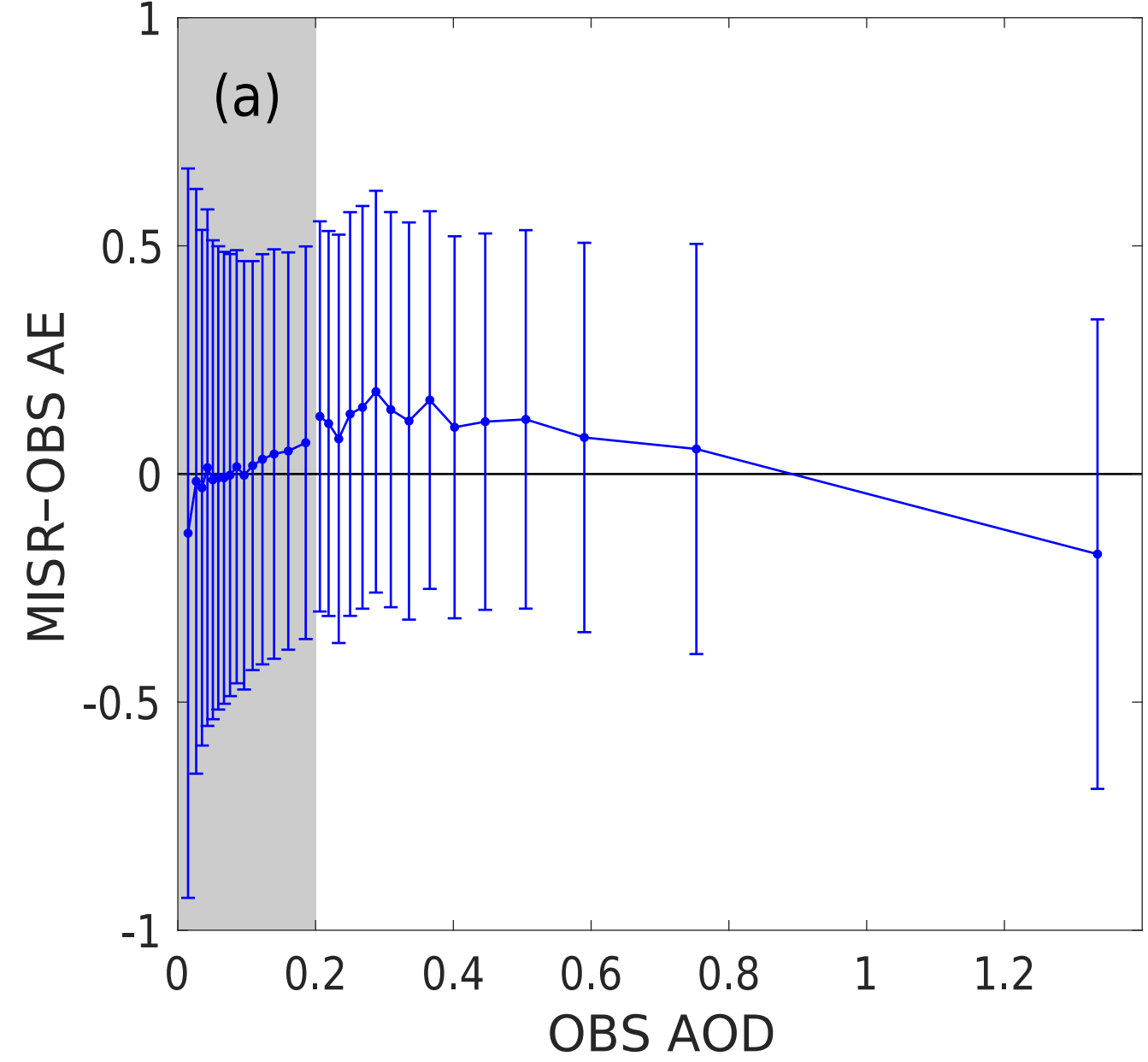
V22 AE error vs. AOD
