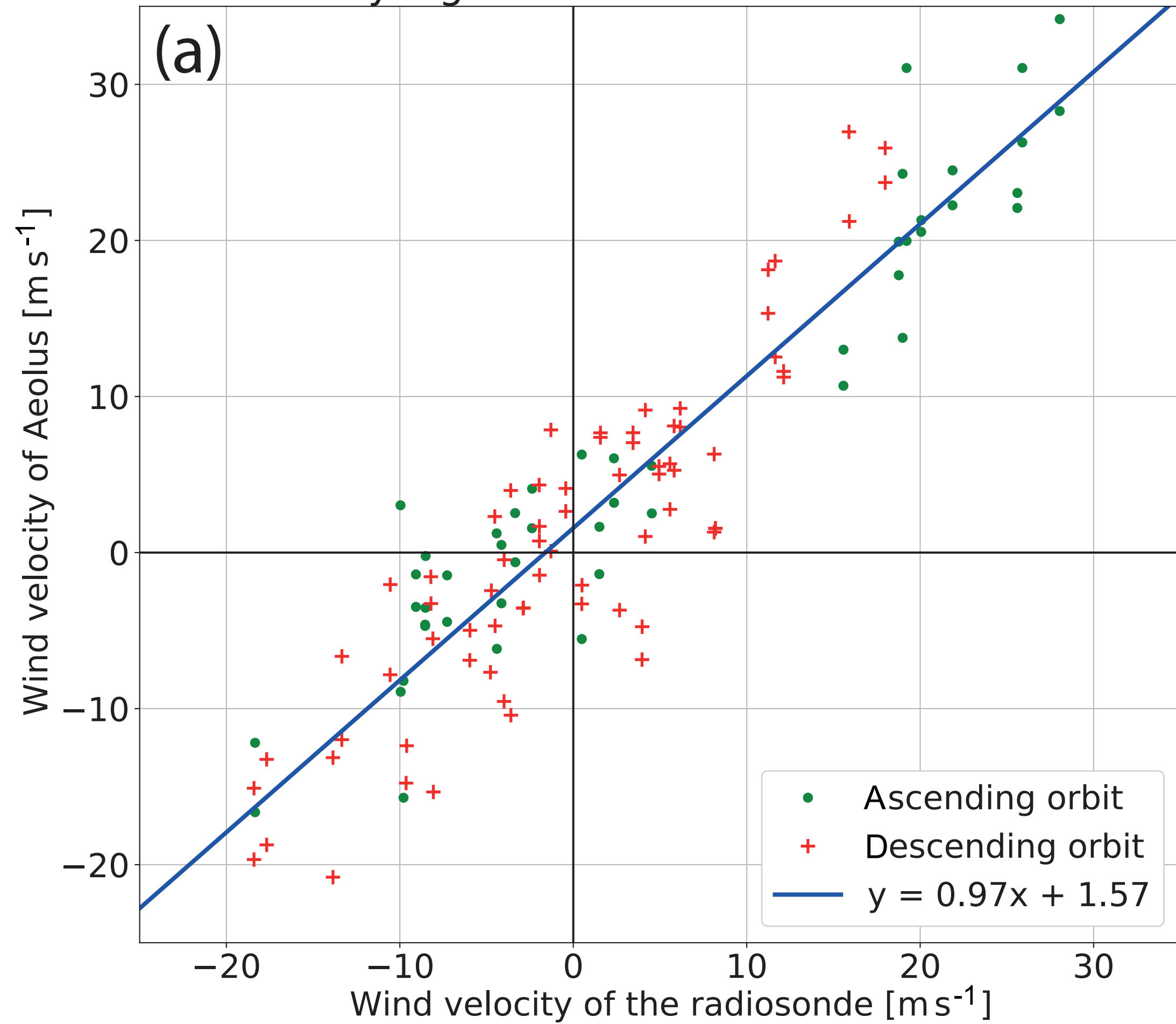
Rayleigh L2B wind vs. radiosonde
