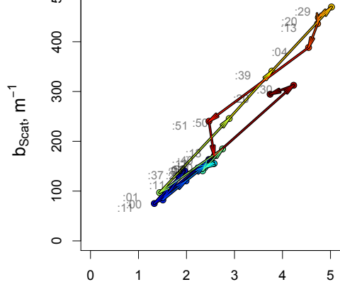
(d) Diagnosed MERET C_{\text{burn}} , ppm
