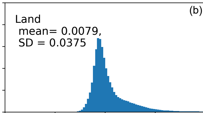
S5P minus OMI
