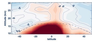
(c) Aer_{gt\ 0.3} - Aer_{lt\ 0.3} (997 nm)
