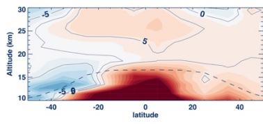
(a) Aer_{gt\ 0.3} - Aer_{lt\ 0.3} (745 nm)
