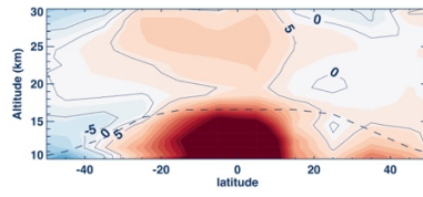
(b) Aer_{gt\ 0.3} - Aer_{lt\ 0.3} (869 nm)
