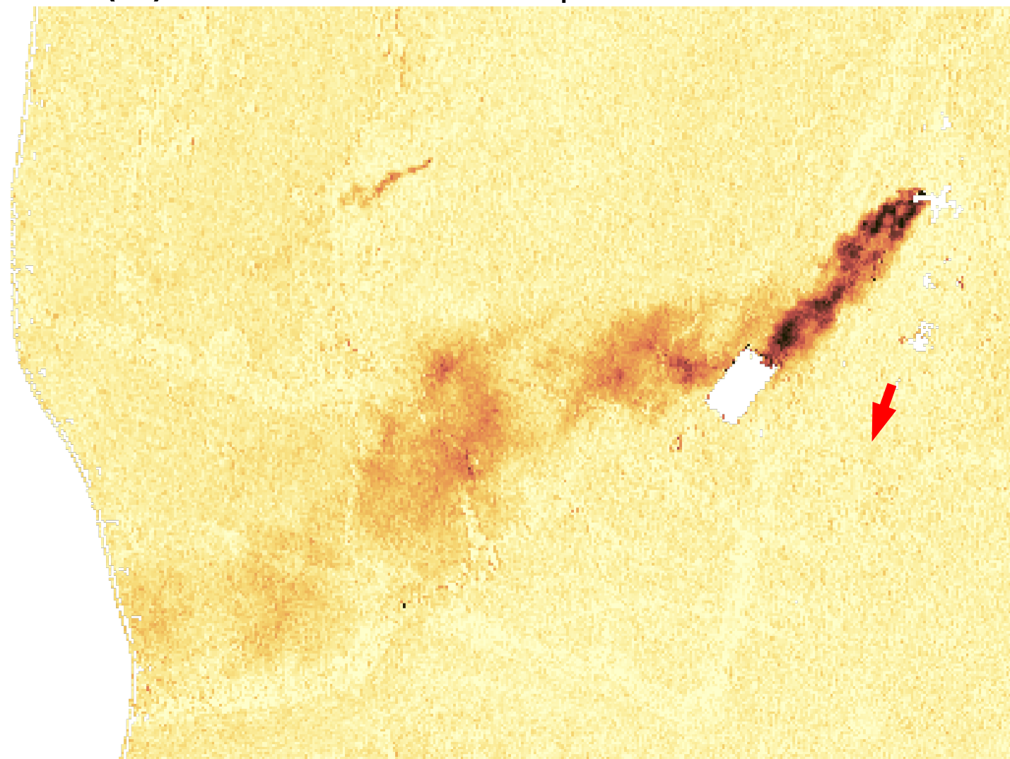
(b) WFM-DOAS CH 4 enhancement
