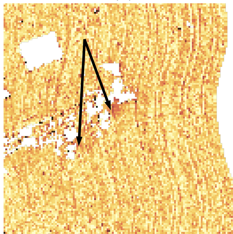
CH 4 enhancement
