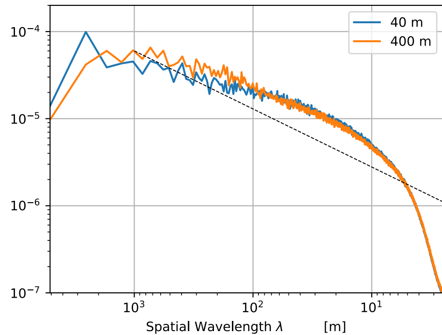
(d) Horizontal wind speed U
