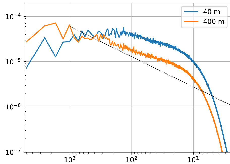
(d) Horizontal wind speed U
