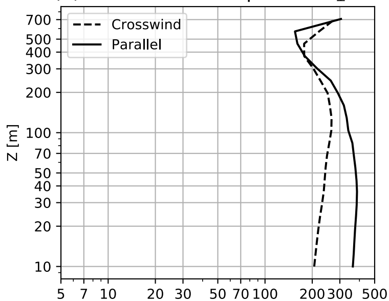
(d) Horiz. Wind Component U_{\perp}
