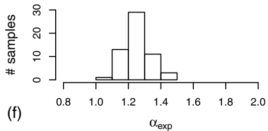
AE31_4 \lambda _C PaM
