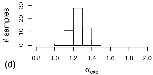
AE31_4 \lambda _C PP
