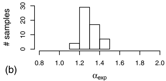
AE31_4 \lambda _C 0
