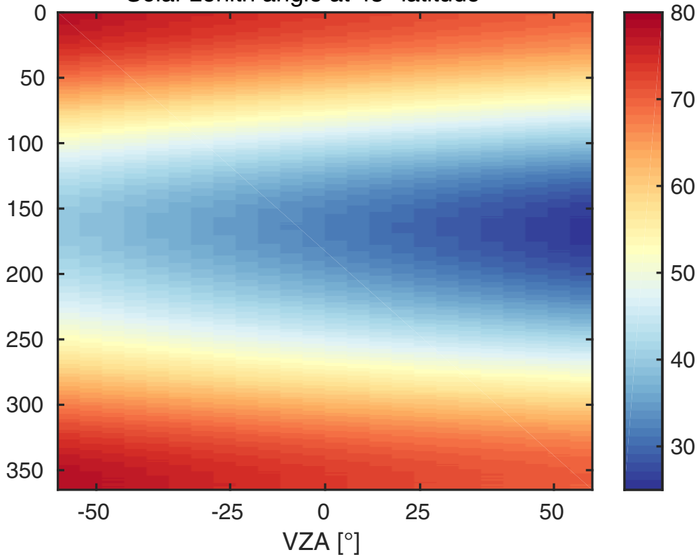
Solar zenith angle at 45° latitude
