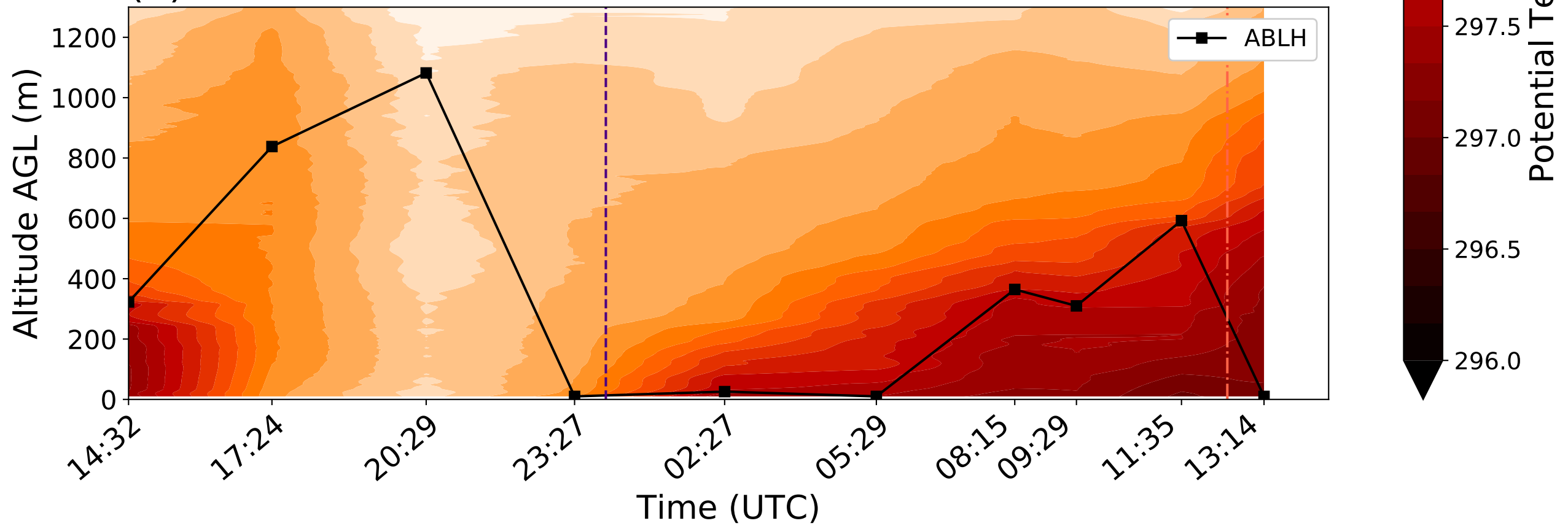
(b) Radiosonde
