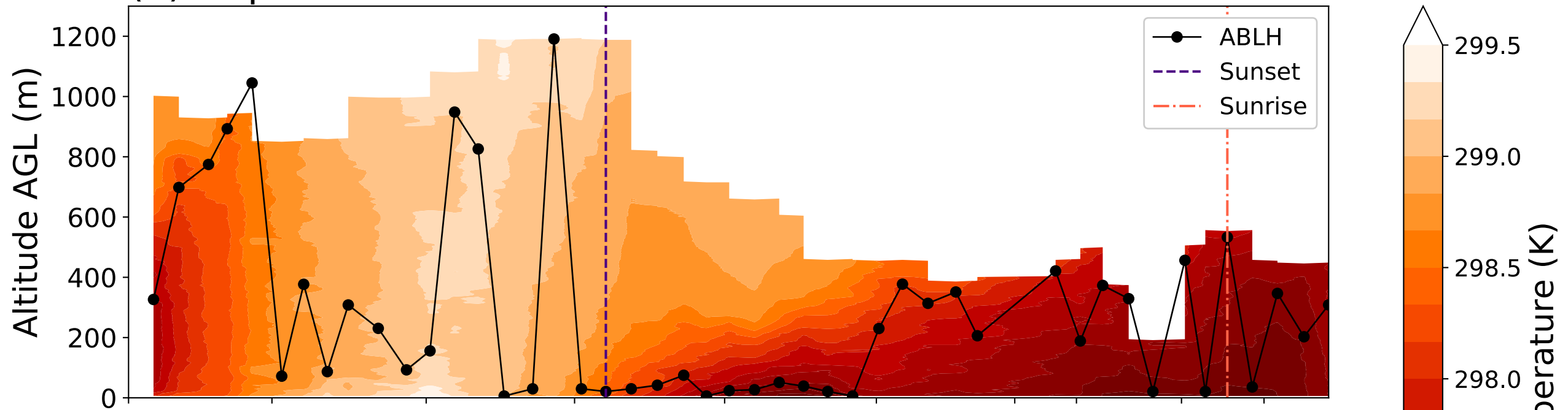
(b) Radiosonde
