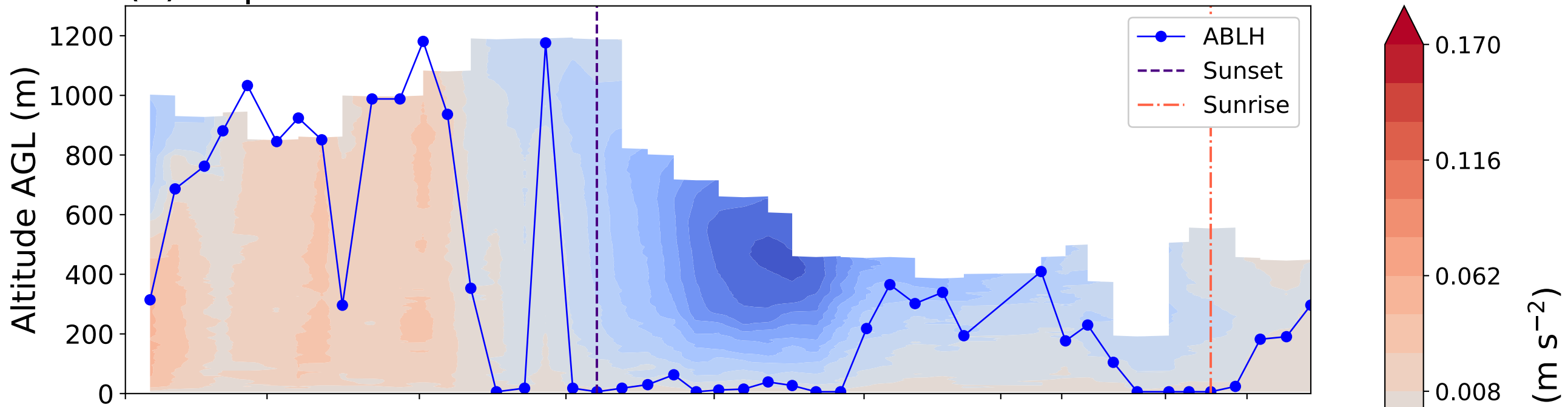
(b) Radiosonde
