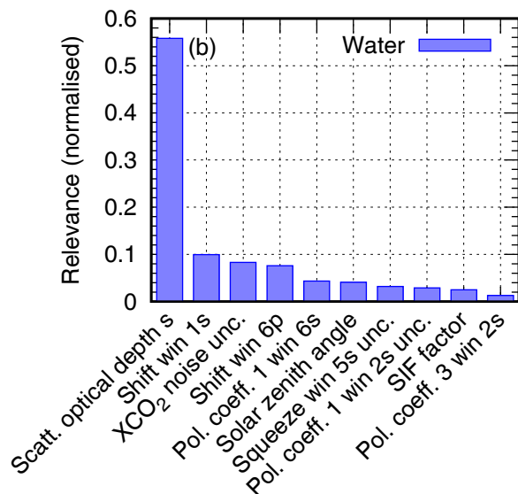
GOSAT XCO2
