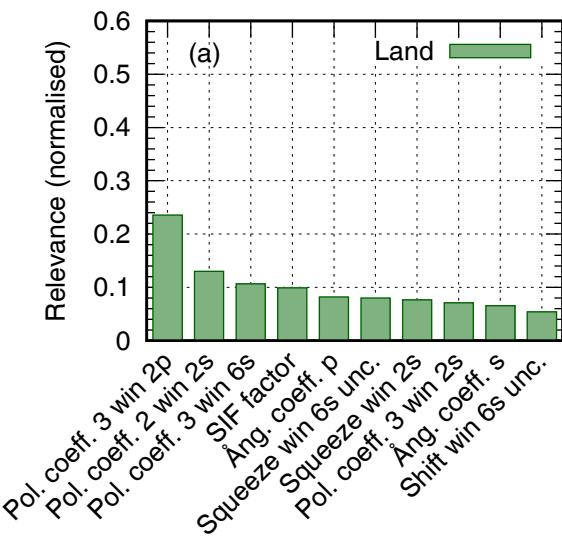
GOSAT XCO2
