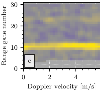
MRR-PRO 23
