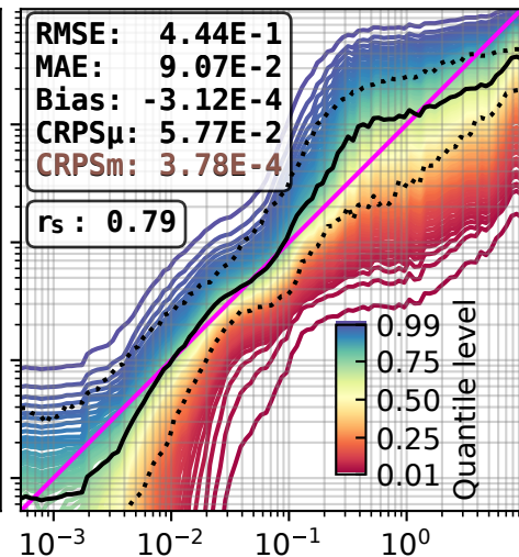
IR
