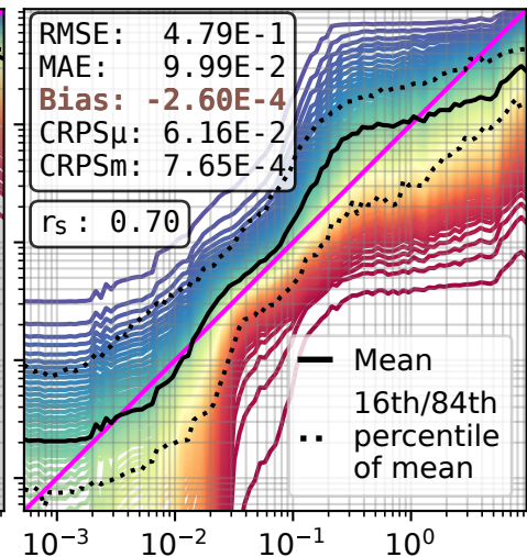
IR subset
