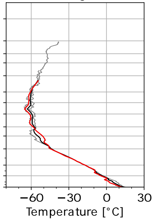
(b) MA:Nighttime
