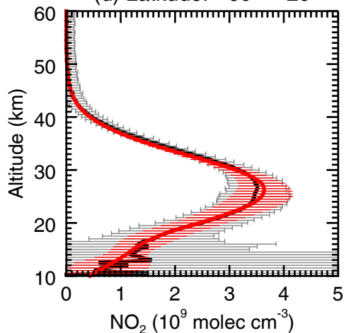
(d) Latitude: -60^{\circ} - -20^{\circ}
