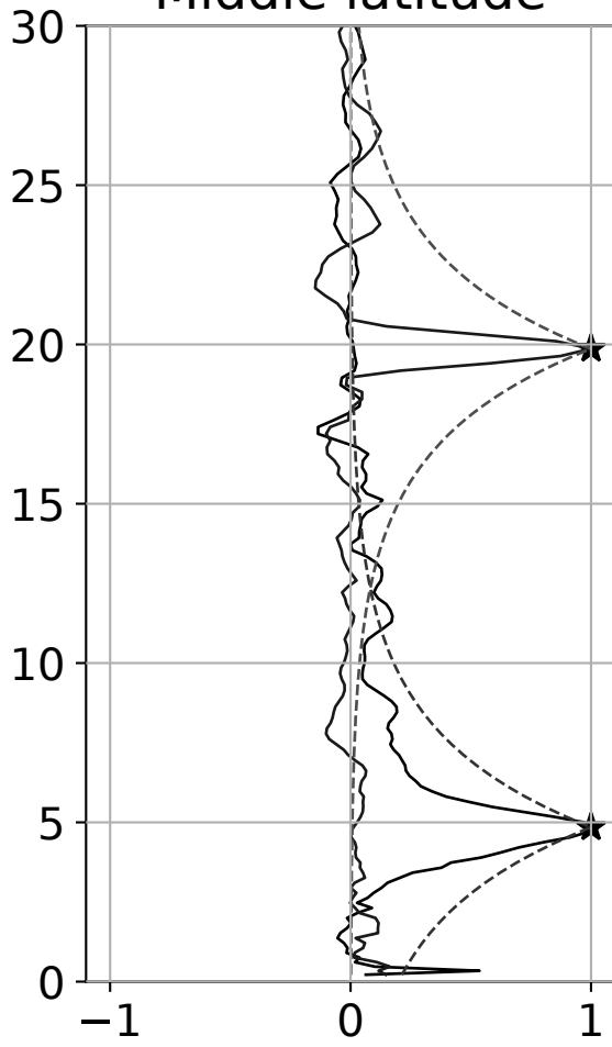
Middle latitude
