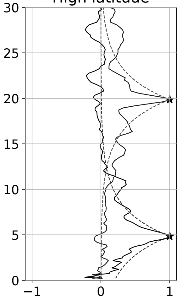
High latitude
