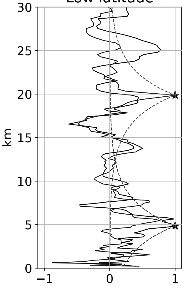
Low latitude
